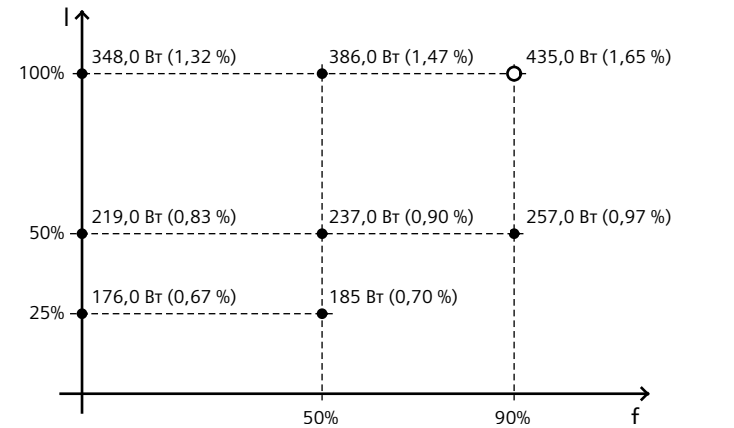
Значения в процентах указывают потери относительно номинальной кажущейся мощности преобразователя. The percentage values show the losses in relation to the rated apparent power of the converter.
